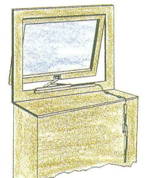
PRIMAT-A - ulospäin aukeava ikkuna - joustavalla tangolla - ikkunassa smyygi
